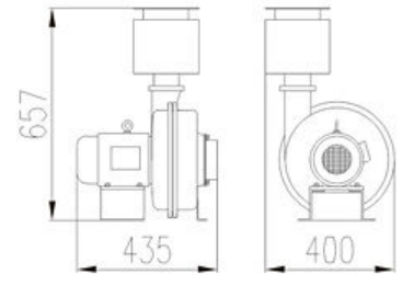
Blower B-200
