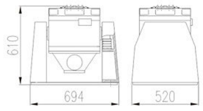
Shaker ET-2-150
