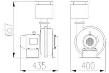
Blower B-200
