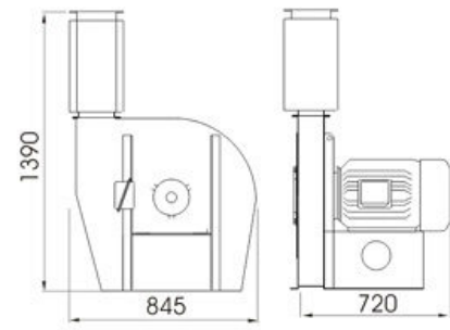
Blower B-3000
